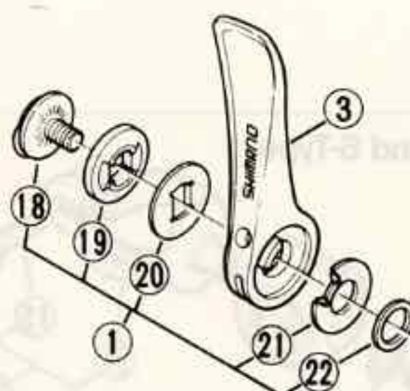
Brazed-on A-Type
