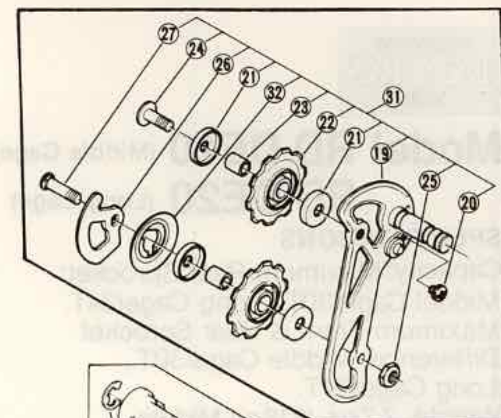
Long Cage
