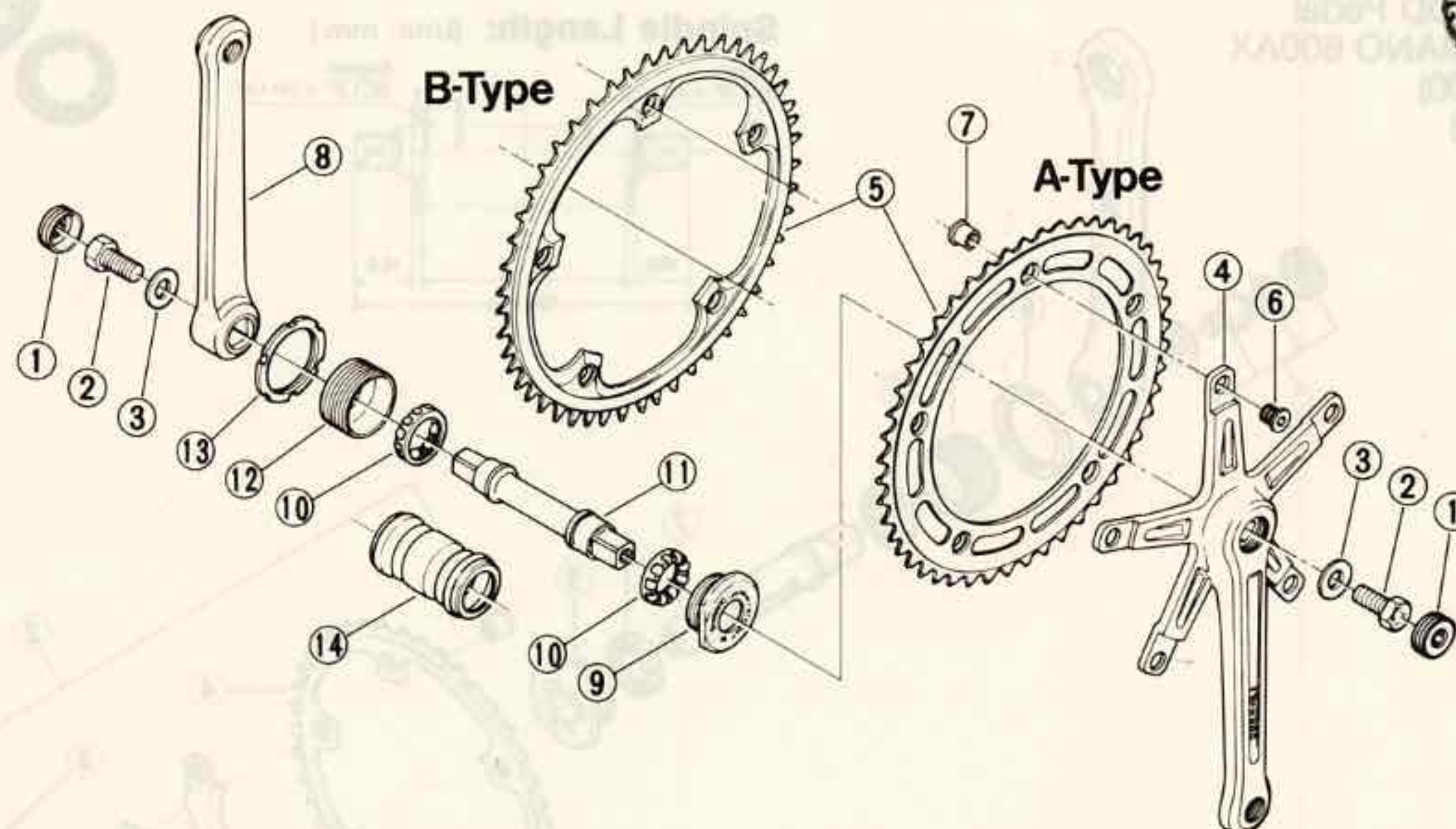
A-Type Gear
